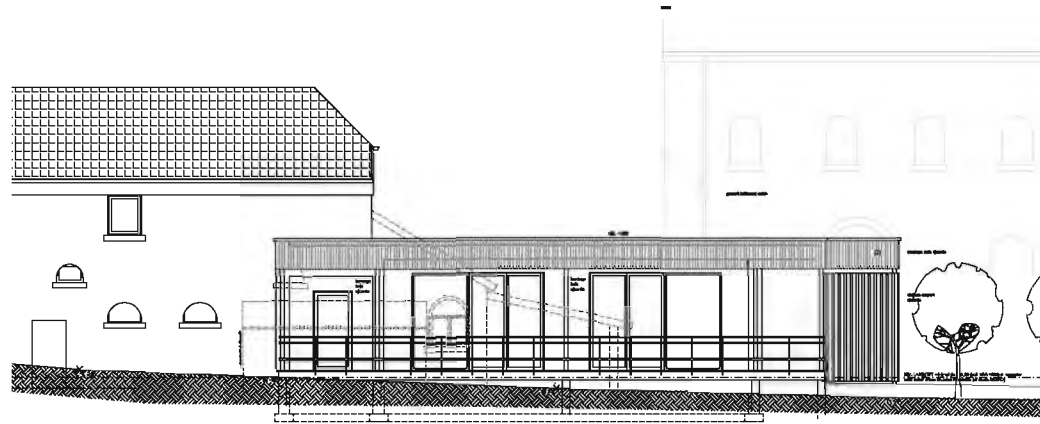
FACADE SUD-EST (1/50)
