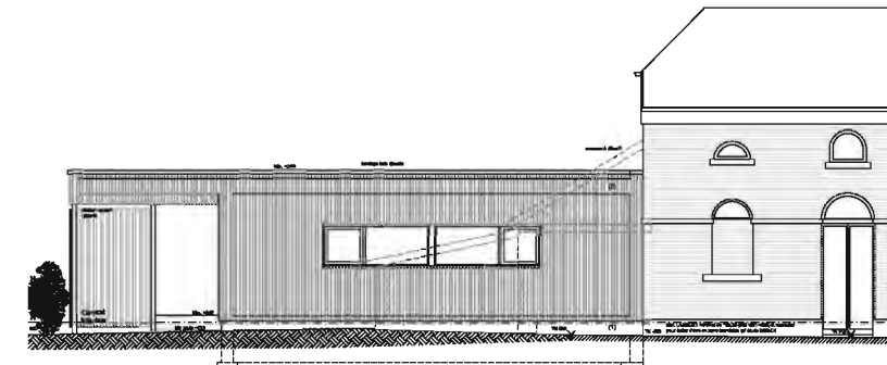
FACADE NORD-OUEST (1/50)
