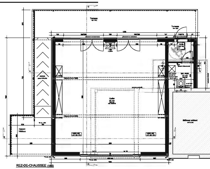
REZ-DE-CHAUSSEE (1/50)
