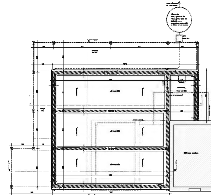
FONDACTIONS (1/50)
