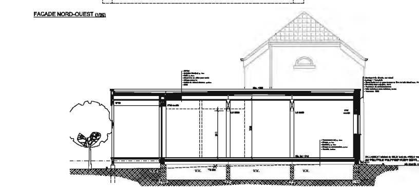
COUPE CC (1/50)
