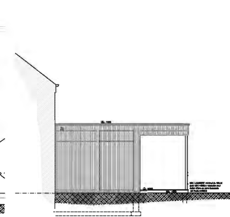
FACADE SUD-OUEST (1/50)
